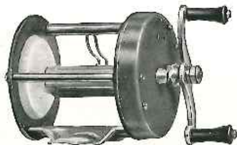
Art. 317 - Da lancio quadruplicatore (rapporto di recupero 1 giro di manovella=4 giri della bobina) guidafilo.
